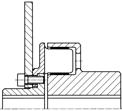
CENTAFLEX-E-3 with brake disc CENTAFLEX-E-3 mit Bremscheibe
